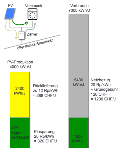
Abbildung 3: 4kWp Anlage-Beispiel B
