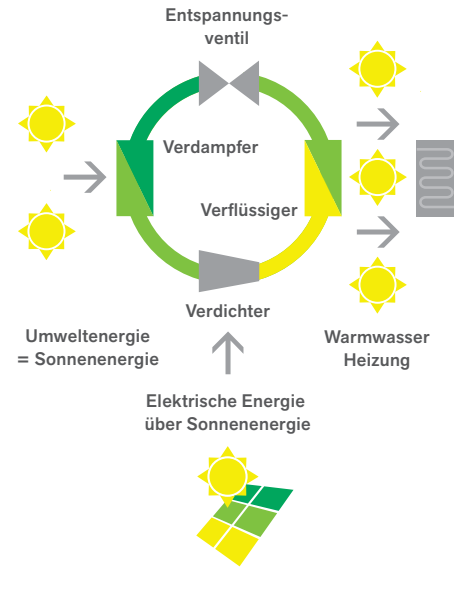
Schematischer Aufbau der Wärmepumpe
